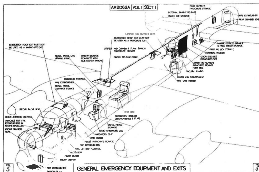
In de opengewerkte tekening van de Lancaster is zichtbaar waar het seinpistool werd opgeborgen (Signal Pistol Stowage), waar men de lichtkogels bewaarde (Signal Pistol Cartridge Stowage) en is de opening te zien waar men door omhoog schoot (Signal Pistol MTG Upward Firing).
